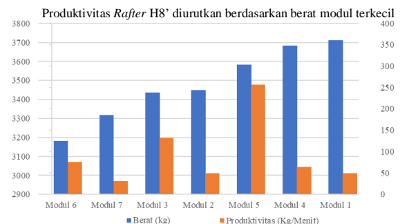
Gambar 12. Berat dan Produktivitas Rafter H8'
