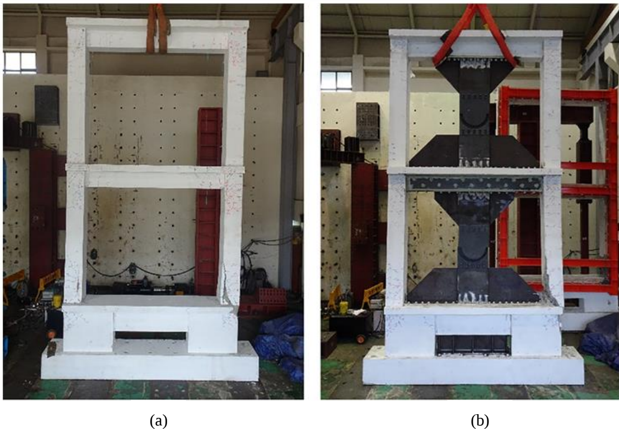
Gambar 1. Spesimen uji rangka beton bertulang dua lantai (Eskandari Nasab et al., 2021).
