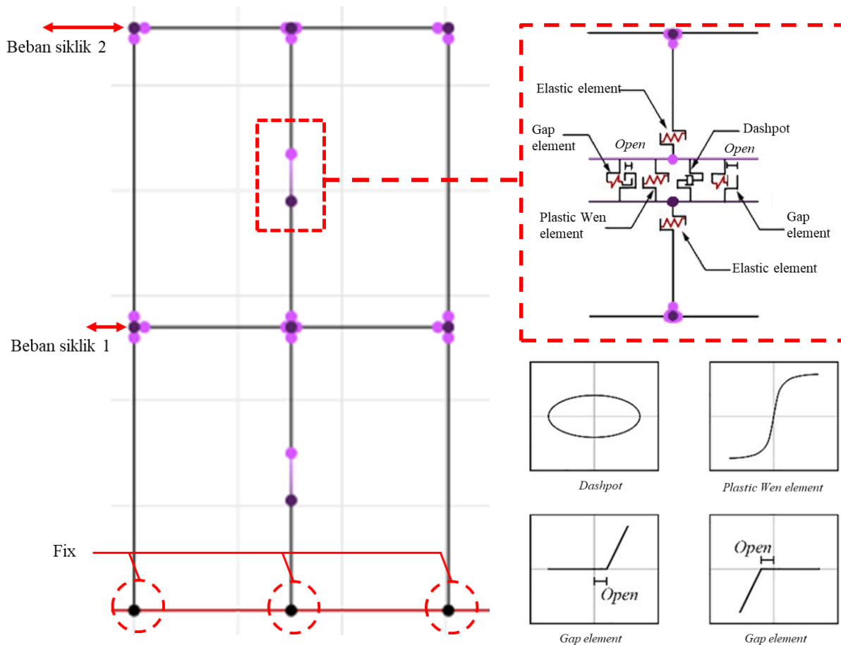
Gambar 3. Model numerik struktur beton bertulang 2 lantai dan analisis model VED.
