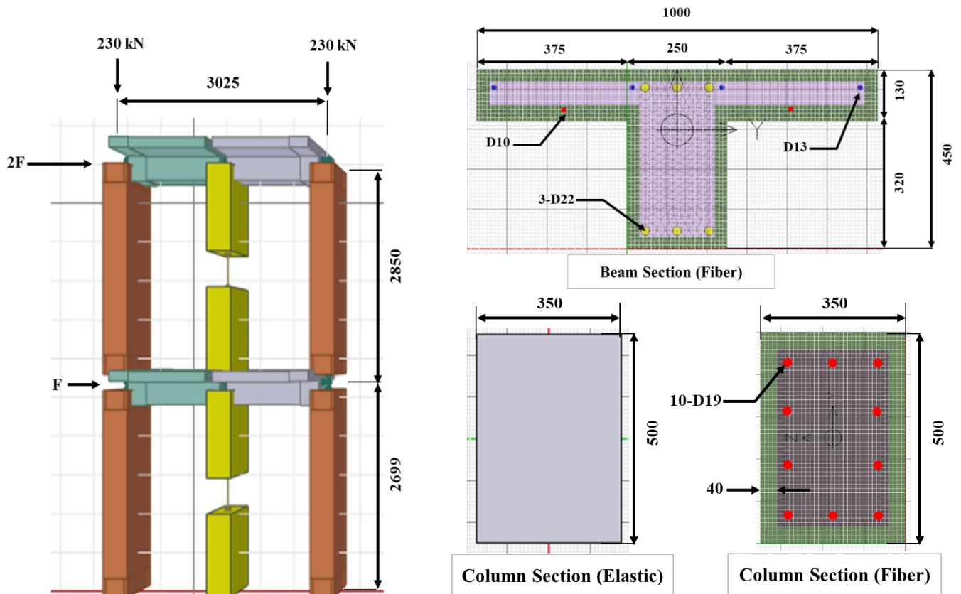
Gambar 2. Detail geometri spesimen uji rangka beton bertulang dua lantai.
