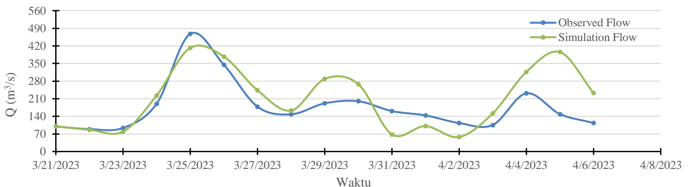
Gambar 4. Hidrograf dengan parameter awal
